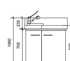
Attentes plomberie
