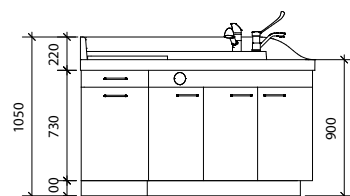
Attentes plomberie
