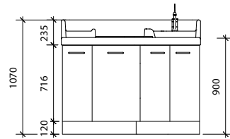
Attentes plomberie
