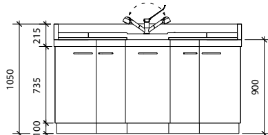
Attentes plomberie
