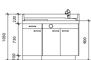
Attentes plomberie
