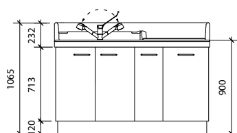
Attentes plomberie
