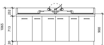
Attentes plomberie
