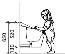
Attentes plomberie
