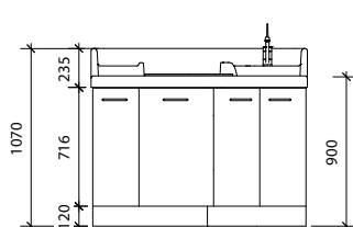
Attentes plomberie
