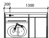
Attentes plomberie
