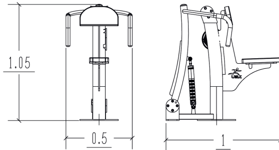
Station d'exercice à charge réglable.
